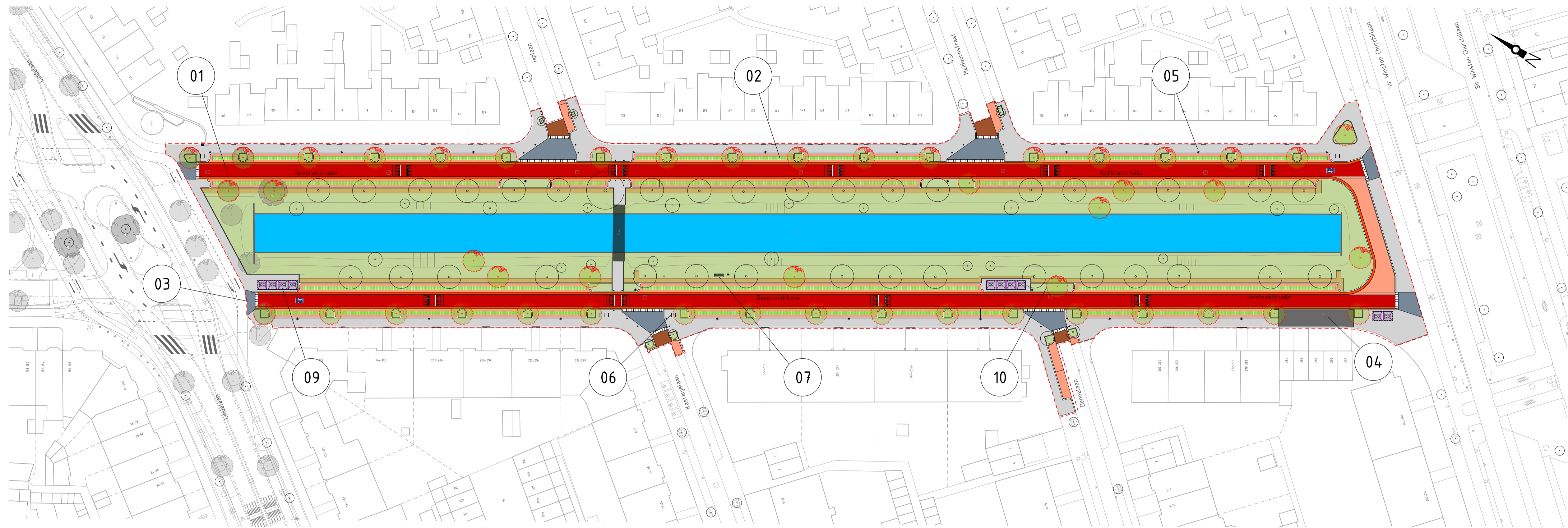
01. Fietsstraat asfalt met rabatstrook
