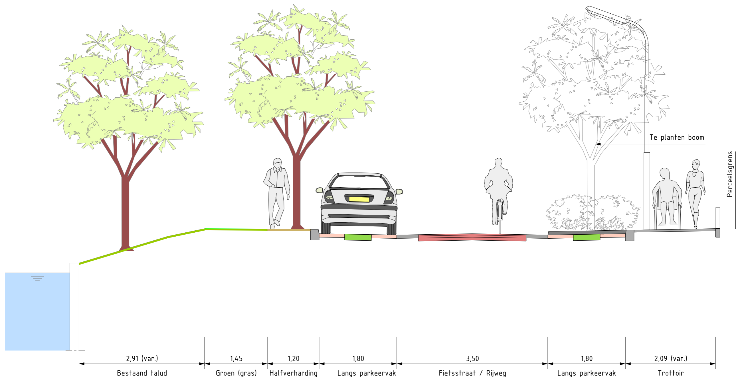
Dwarsprofiel 02 Nieuwe situatie SCHAAL 1 : 50
